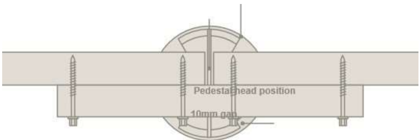
Bild 5. In die Verbindungsstücke 8 mm Löchern bohren und mit etwas Spiel verschrauben (Schrauben nicht satt anziehen) und zwischen den Längsstössen mindestens einen Spalt von 10 mm lassen
