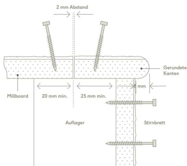
Der Überhang des Abschlusses darf max. 8 mm betragen
